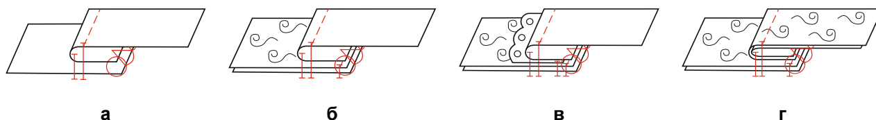
Рисунок 1 – Варианты технологических решений однослойного сборочного комплекса различной слойности: а – слойность 1/1; б – слойность 2/1; в – слойность 3/1; г – слойность 2/2
