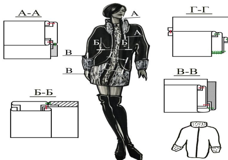
Рис. 1 Конструкторско-технологическое решение процесса изготовления женской шубы из искусственного меха. - сварной шов, - ниточный шов.
