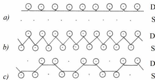
Şəkil 1. Saya (a), lastik 1+1 (b) və lastik 2+2 (c) hörmələrinin qrafik yazılışı
