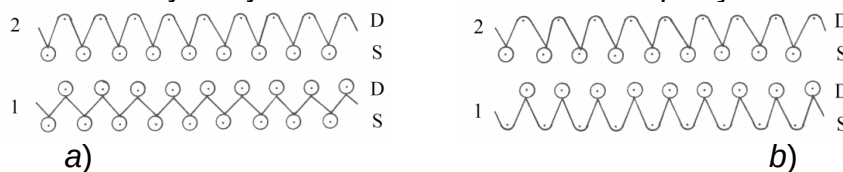
Şəkil 5. İkiqat yarımfanq (a) və fanq (b) hörməli trikotajın qrafik yazılışları
