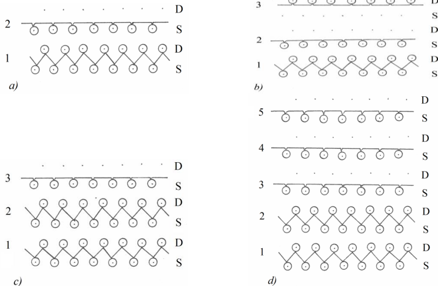
Şəkil 3. Reps (a), Milan lastiki (b) və İsveçrə ilməsi (c) və relyefli lastik (d) hörmələrindən alınan trikotajın qrafik yazılışları
