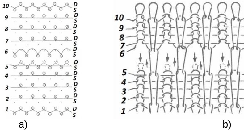
Şəkil 4. Kuponun ayırıcı sahəsinin qrafik yazılışı (a) və quruluşu (b)
