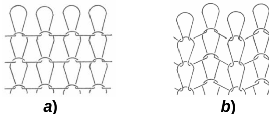
Şəkil 2. Saya (a) və lastik 1+1 (b) hörmələrinin qrafik yazılışına uyğun çəkilmiş quruluşu
