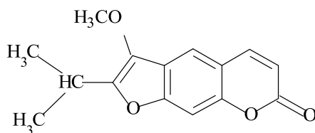
Peysedanin
