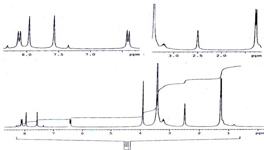
Şəkil 2. Peysedanin kumarin törəməsinin ^1\text{H} NMR-spektri
