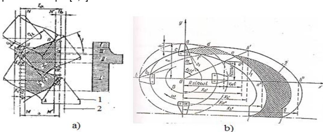
Şəkil 1. Kövşənin kəsilmə hündürlüyü diaqramı: a-dayaqlı kəsilmədə; b-dayaqsız kəsilmədə Seqmentli-barmaqlı kəsən aparatlar aşağıdakı həndəsi və kinematik parametrlərlə xarakterizə olunurlar:
