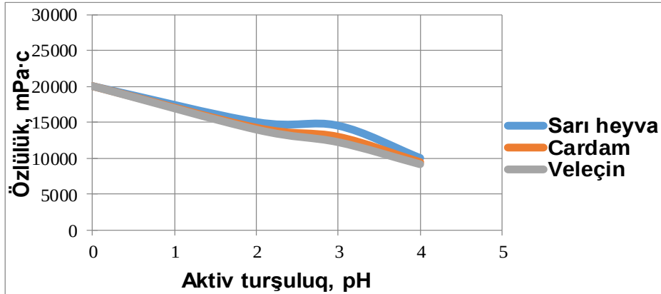
Şəkil 1. Kappa-karraginanla işlənmiş heyva jelesi üçün özlülüyün aktiv turşuluqdan asılılıq qrafiki
