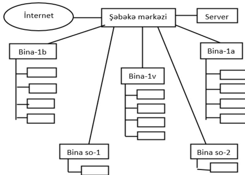
Şəkil 2. Çox saylı binalar üçün Strukturlaşdırılmış kabel sisteminin məntiqi quruluşu
