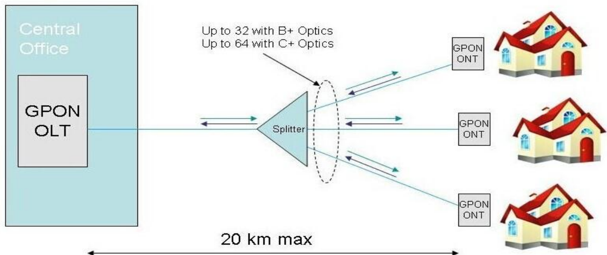
Şəkil.1. Gpon texnologiyası.
