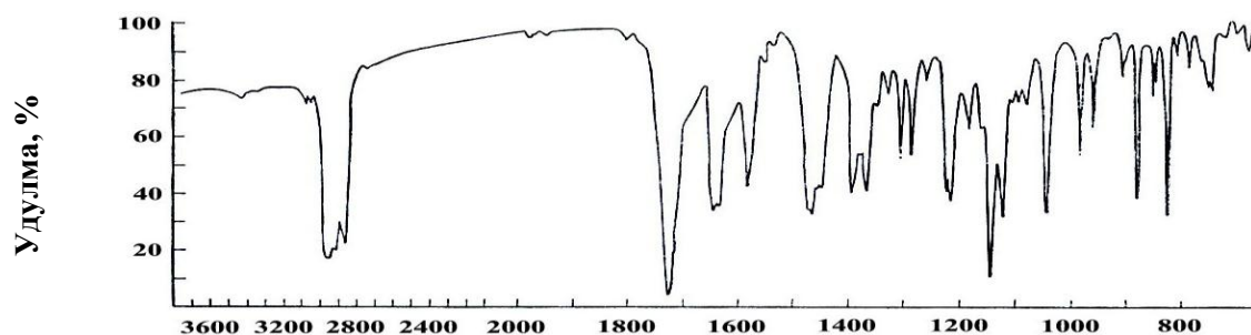
Şəkil 1. Peysedanin kumarin törəməsinin İQ-spektri
