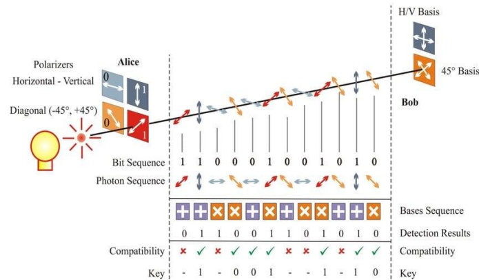
Şəkil 1. BB84 protokolunun işləmə arxitekturası
