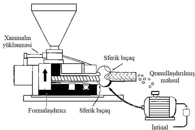
Şəkil 1. Sferik bıçağı olmayan pres-ekstruderin işləmə sxemi.
