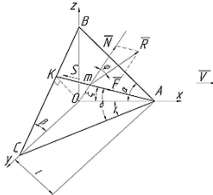
Şəkil 1. Pazın döşəmə materialı ilə təmas sxemi.
