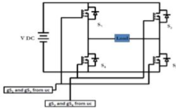
Şəkil 2. Tam bir fazlı H-körpü invertoru.
