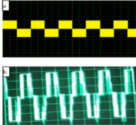
Şəkil 7. Signalın modelləşdirilməsi (a) və eksperimental signalın nəticələri (B) tam tək fazlı inverterin signal formasının çıxış forması
