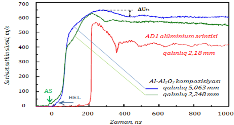
Şəkil 1. Tədqiq olunan kompozitlərin və texniki təmiz AD1 alüminium ərintisinin sərbəst (arxa) səth sürəti profillərinin müqayisəsi.
