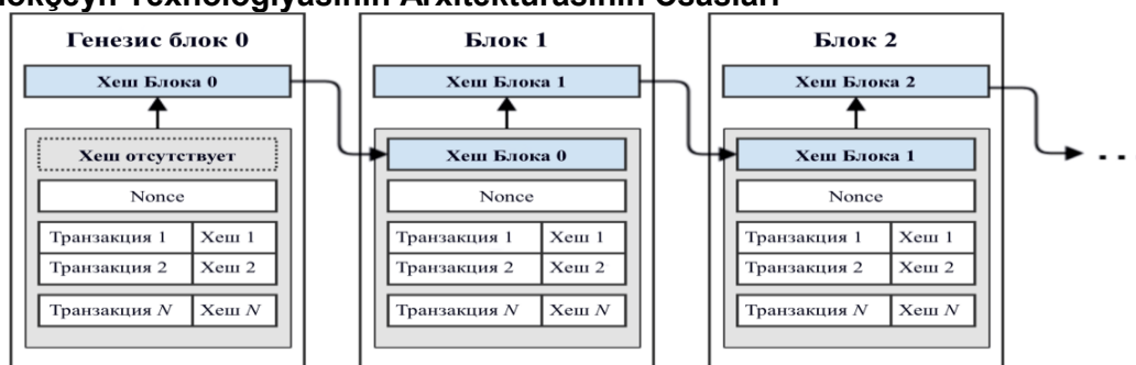
Şəkil 1. Blokların ardıcılığı və blokçeyn şəbəkəsi
