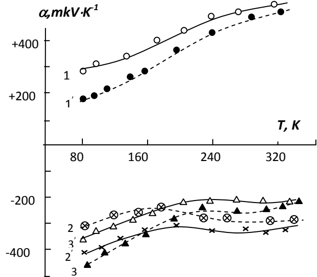
Şəkil 2. Termo.e.h.q - \alpha , temperatur asılılığı 1-SnSe; 2- Sn_{0,99}Tb_{0,01}Se , 3- Sn_{0,95}Tb_{0,05}Se . 1', 2' və 3' -şüalanmadan sonra
