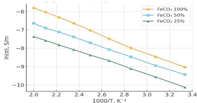
Рис. 1. Зависимость \ln(\sigma) от 1000/T для различных композитов \text{FeCO}_3 –бентонит.
