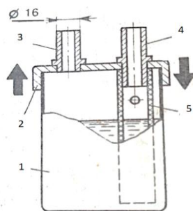
Схема барботера
