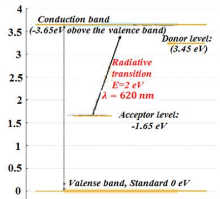
Şəkil 4. ZnS kristallarının sxematik zona diaqramı
