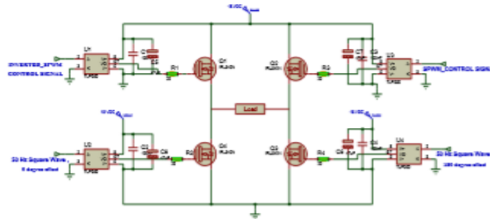
Şəkil 6. Tam N-körpü və ötürücü zəncirlərinin prinsipial sxemi
