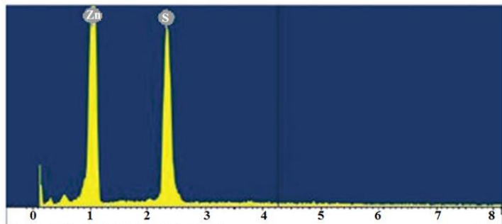
Şəkil 2. ZnS kristallarının səthinin rentgen mikroanalizi
