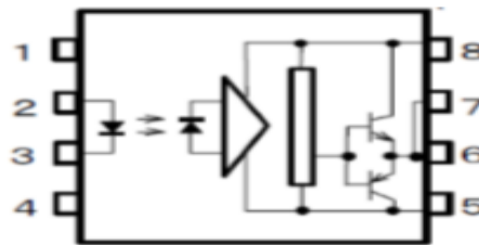
Şəkil 5. TLP250 sürücü qapıları
