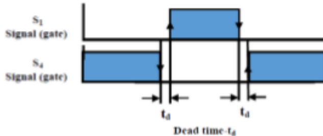
Şəkil 3. Ölü vaxt müşahidəsinin müvəqqəti diaqramı.
