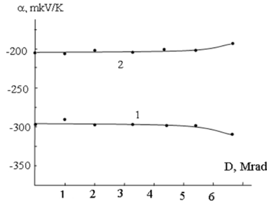
Şəkil 1. Sn_{1-x}Tb_xSe sistem ərintilərdə termo.e.h.q şüalanma dozəsindən asılılığı. 1- x=0,01 ; 2- x=0,05 , T=300K
