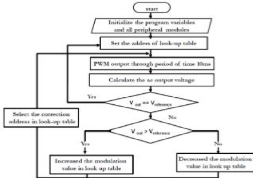
Şəkil 4. Phasoinverter signal SPVM signalinin proqramlaşdırılması üçün blok diaqramı.
