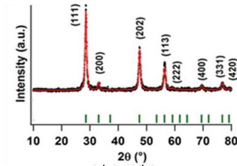
Şəkil 1. ZnS kristallarının rentgen difraktoqramı
