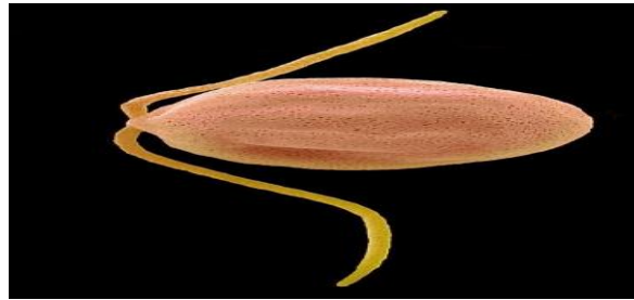
Şəkil 1. Dunaliella salina yosunları
