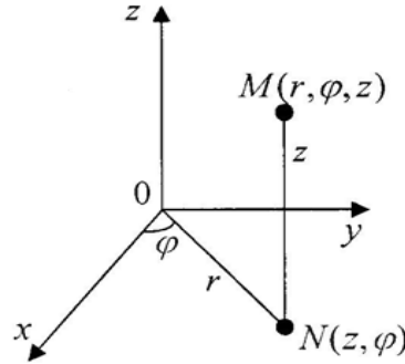
Şəkil 1. Silindrik koordinat sistemi
