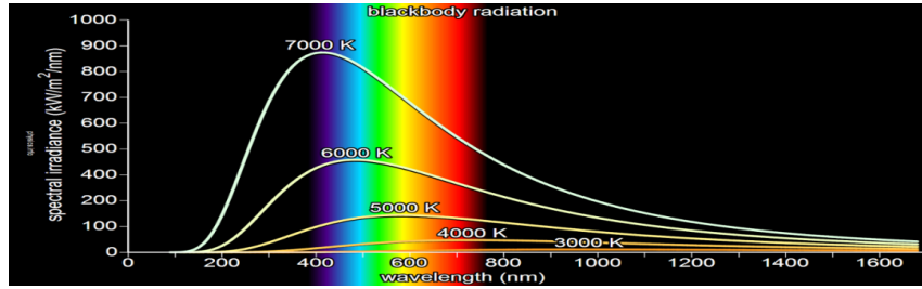
Qrafik 1. Günəşdən gələn ən yüksək enerji diapozonu
