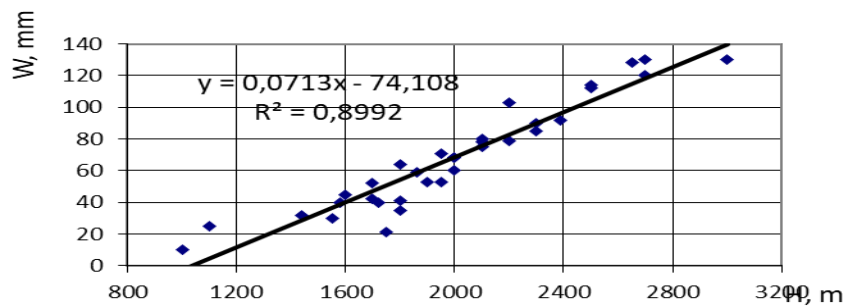
Şəkil 1. Qar örtüyündə sululuğun yerin yüksəkliyindən asılılıq qrafiki (2003-cü il üçün)
